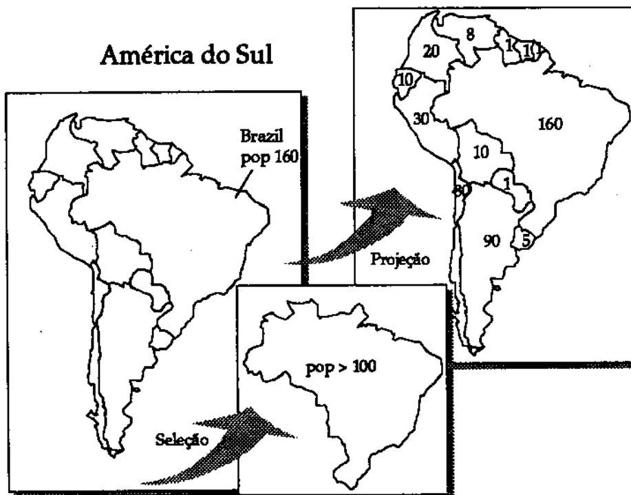
Fig. 4.4 - Projeção Espacial
