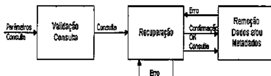
Figura 5.4: Fluxo de dados geral para operações de remoção.
