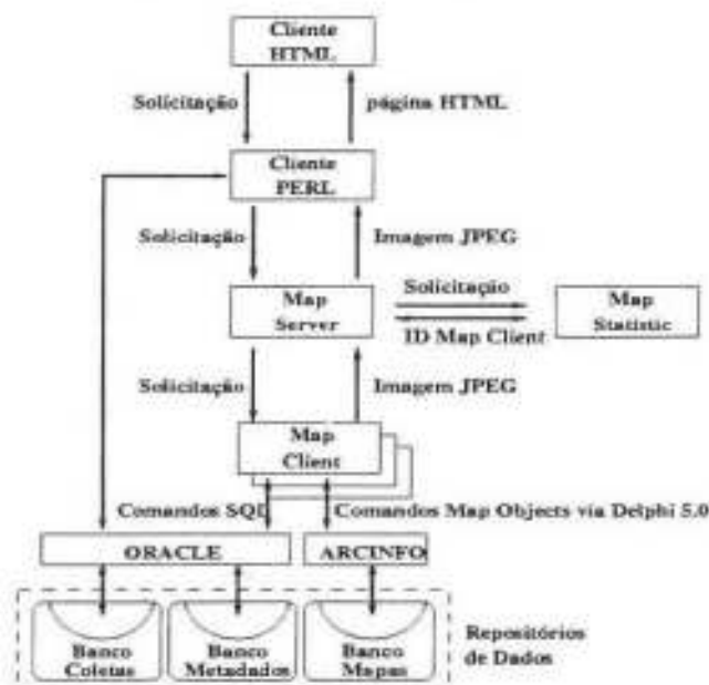
Figura 6.2: Arquitetura do Species Mapper
