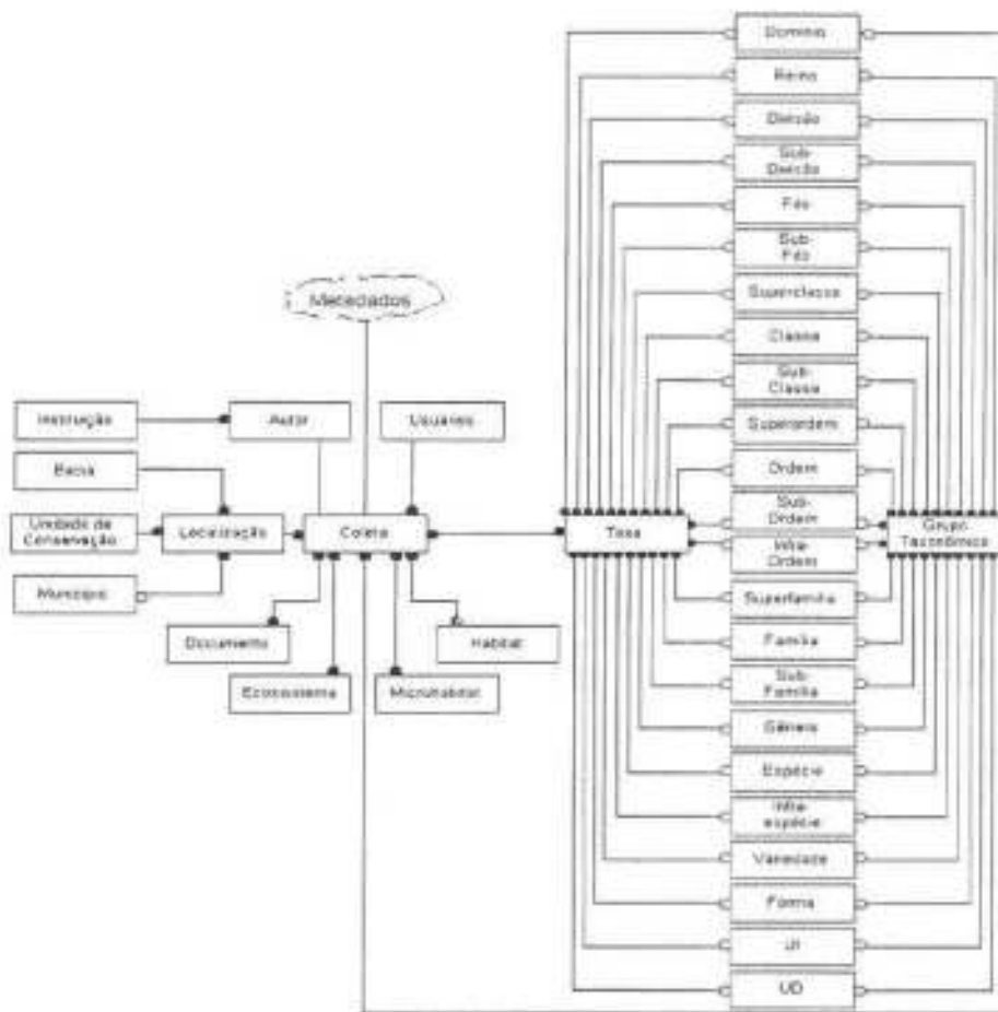
Figura 5.1: Modelagem do Banco de Coletas
