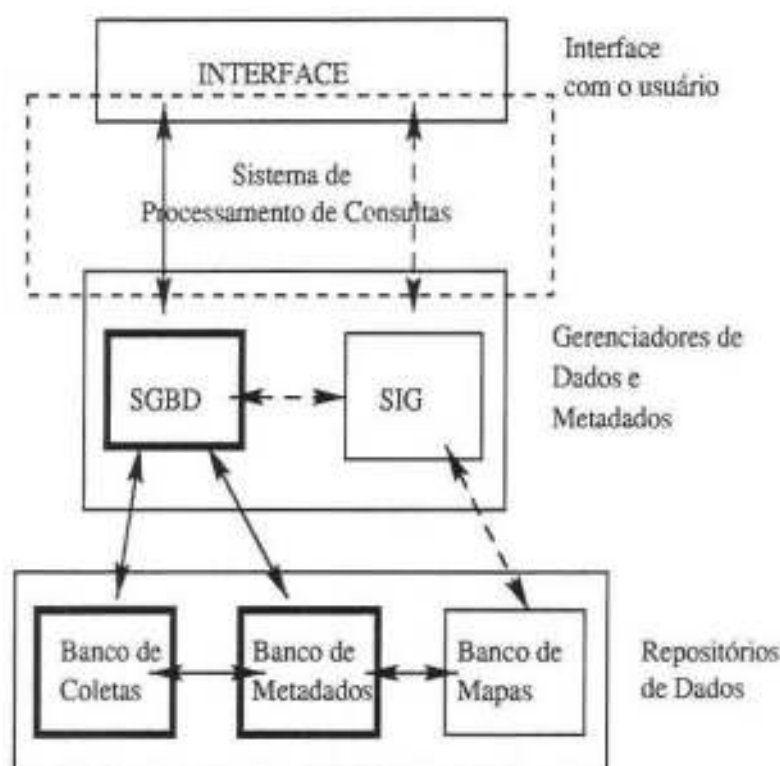
Figura 4.1: Arquitetura básica do SINBIOTASP.
