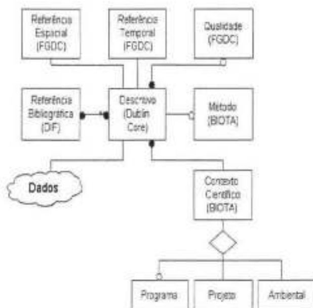
Figura 5.2: Modelagem do Banco de Metadados
